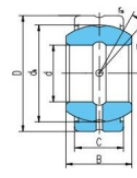
GEZ...ES-2RS
